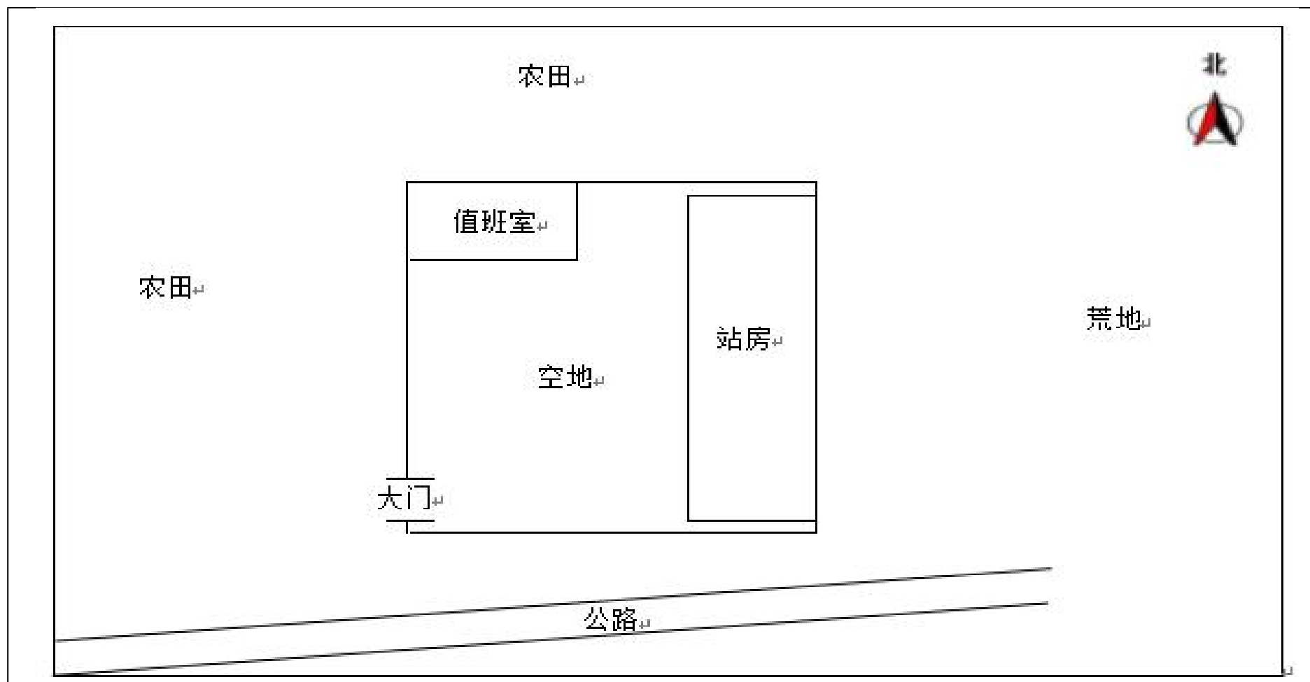
图3 项目平面布置
